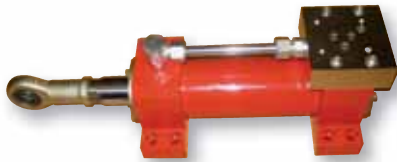
Zylinder mit verstellbarer Schwenkzapfenbefestigung und verdrehbarem Kopf
